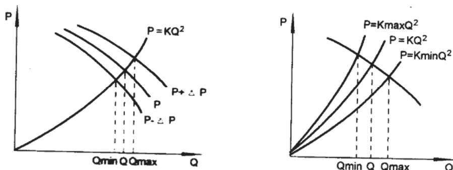
图 2 管网阻力与风机性能关系图
