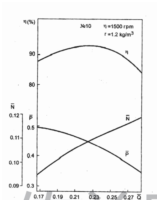
图1 4-68型离心通风机无因次性能曲线
